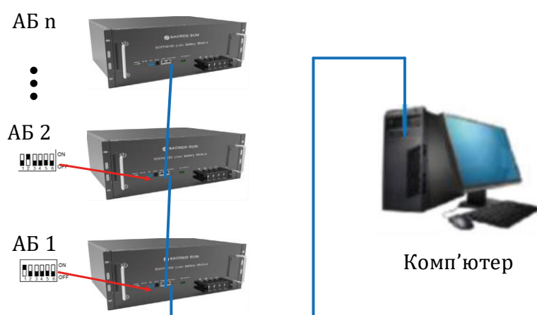
Рисунок 5-2 З'єднання декількох батарей комунікаційним кабелем
