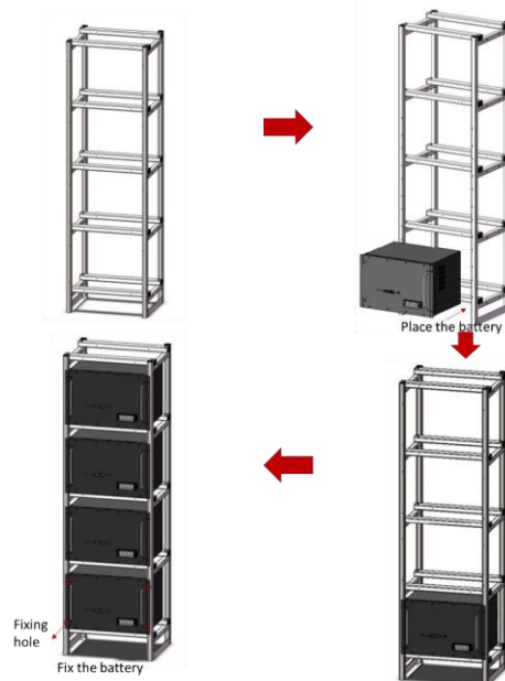
Рисунок 4-1 Встановлення акумуляторів (варіант встановлення)
